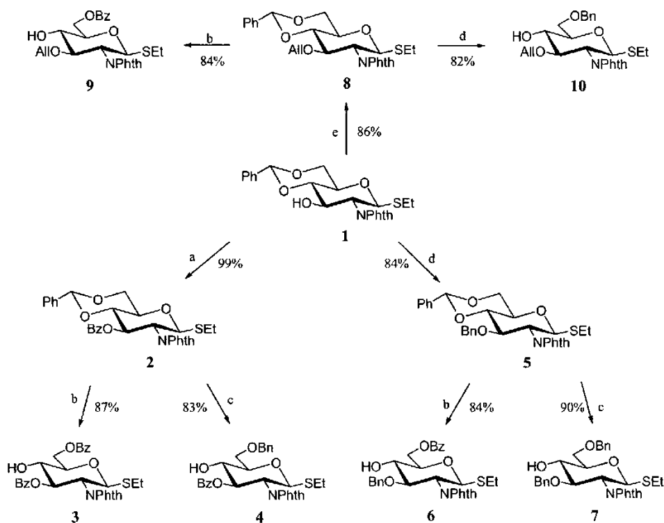
Scheme 2: (a) BzCl, pyridine; (b) 1. ethylene glycol, TFA/CH 2 Cl 2 (5:1); 2. BzCl, pyridine; (c) NaCNBH 3 , Et 2 O/HCl, THF; (d) BnBr, NaH, DMF; (e) AlIBr, NaH, DMF.
